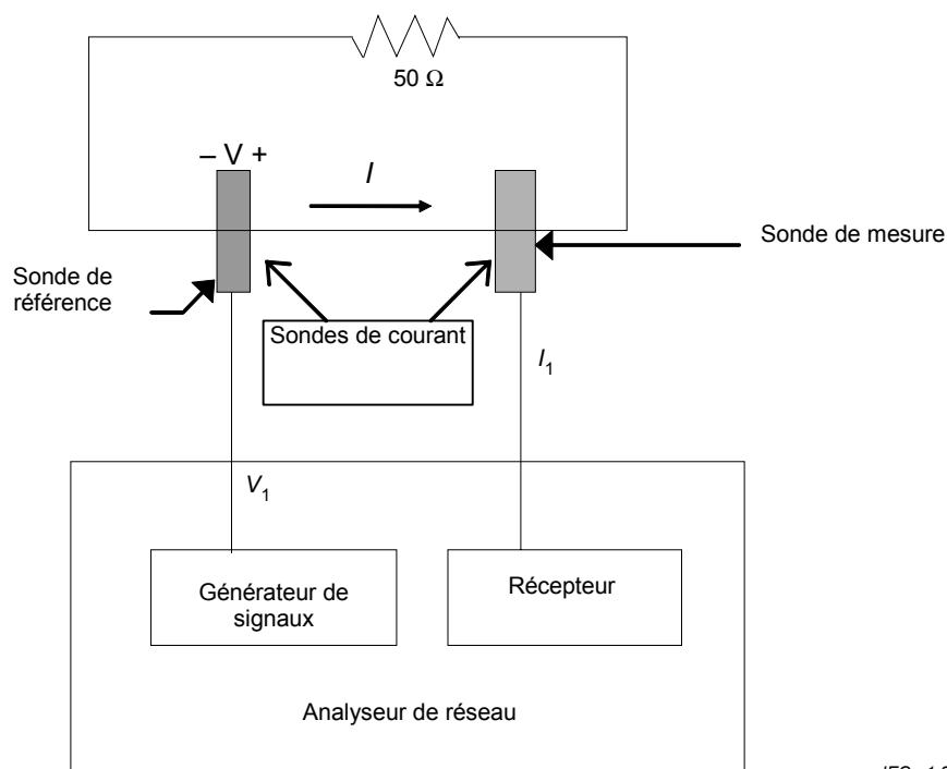
Figure C.4 – Dispositif d'étalonnage
